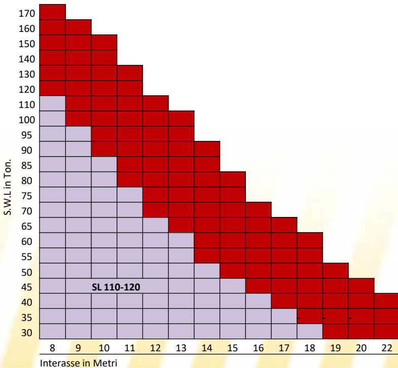
SL 110-120 tabella carico/ Interasse
